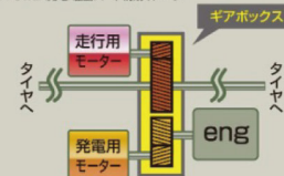
e-POWER発電/駆動(パート構成イメージ)
